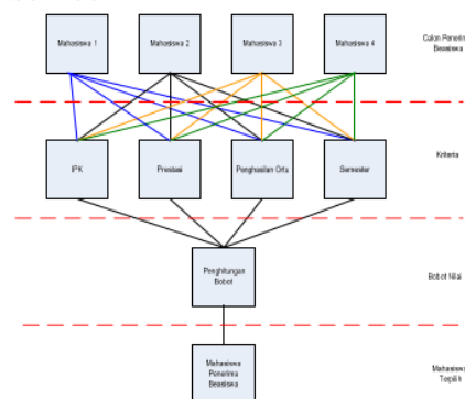
Gambar 1 Hirarki Kriteria Beasiswa
